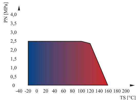
Wykres pola pracy kurka / Pressure-temperature diagram
