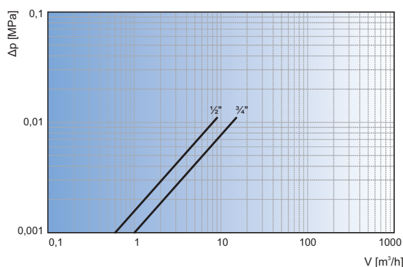
Wykres spadku ciśnienia / Head loss diagram
